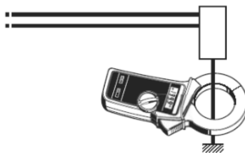
图 4 接地泄漏电流测试
