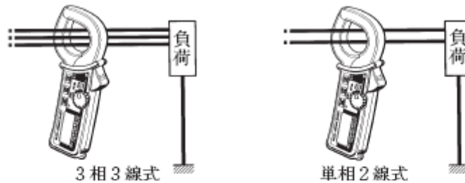
图 2. 零相測定
