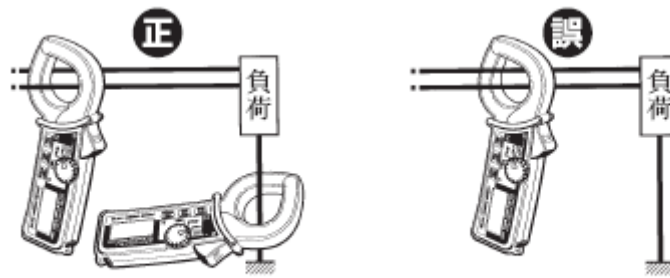
图 1. 通常測定
